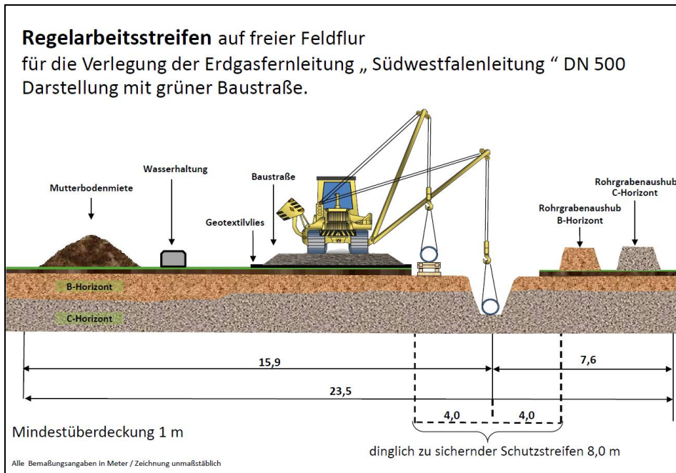
Abb. 2: Schematische Darstellung des Regelarbeitsstreifens auf freier Feldflur DN 500
