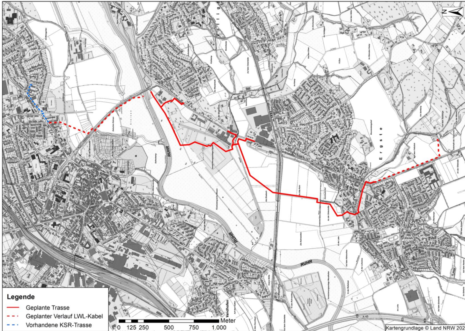
Abb. 1: Übersicht mit geplantem Trassenverlauf
